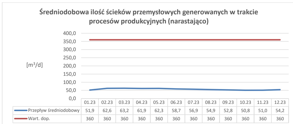
Rys. nr 2. Zmiana średniodobowej ilości dopuszczalnej ścieków przemysłowych (narastająco) odprowadzanych systemem kanalizacji przemysłowej w odniesieniu do ilości dopuszczalnej.
